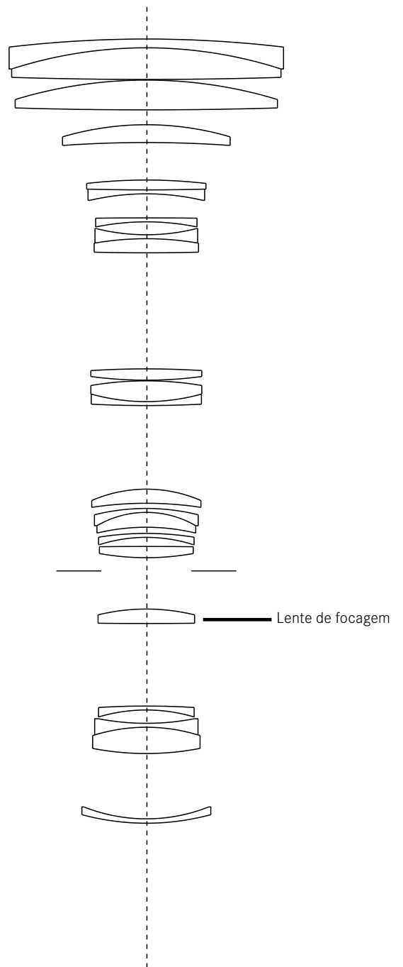
CORTE TRANSVERSAL DA LENTE
