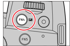
露出補正
