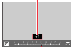
明るすぎる
