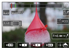
一時停止中
