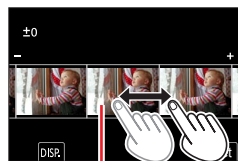
現在の設定
