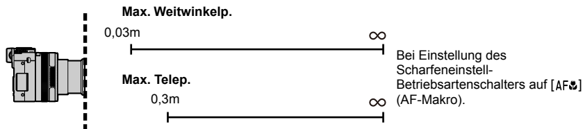
Entfernungs-Einstellbereich
