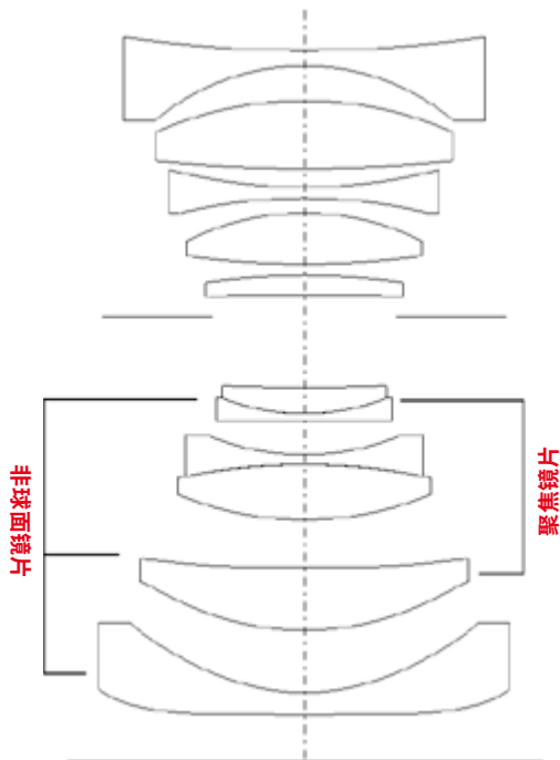
镜头剖面图
