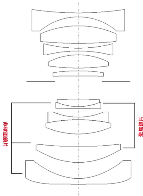
鏡頭剖面圖
